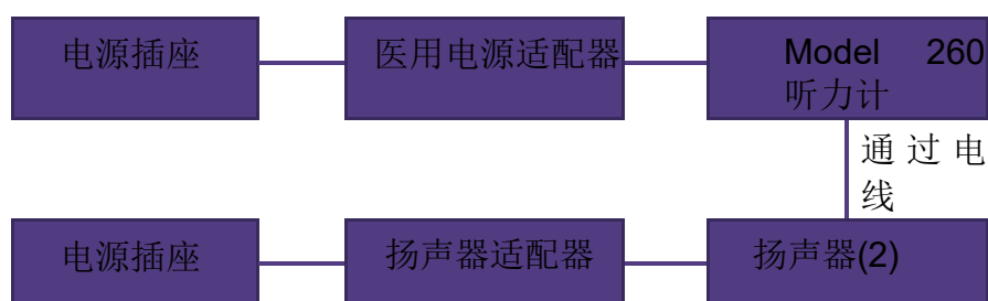
图5: Model 260 听力计与医学认可的电源适配器和外置扬声器一起使用
